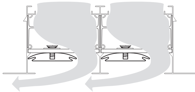
HORIZONTAL DISCHARGE 1 WAY
